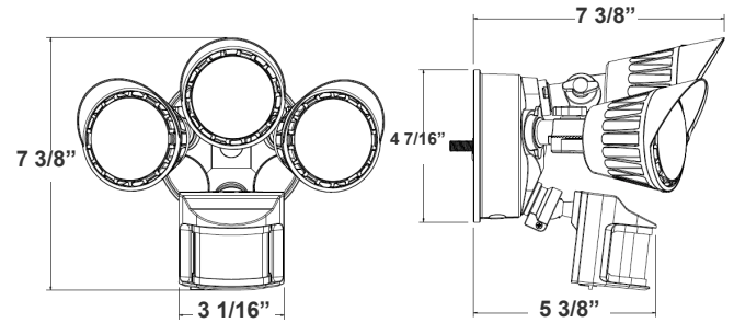
7 3/8" (W) x 7 3/8" (H) x 5 3/8" (D)
