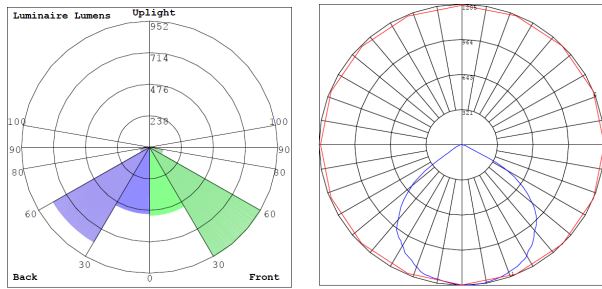
BUG Rating: B2-U1-G0
